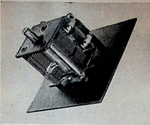
Fig. 2 Afstemcondensator voor gebruik met gedrukte bedrading.
