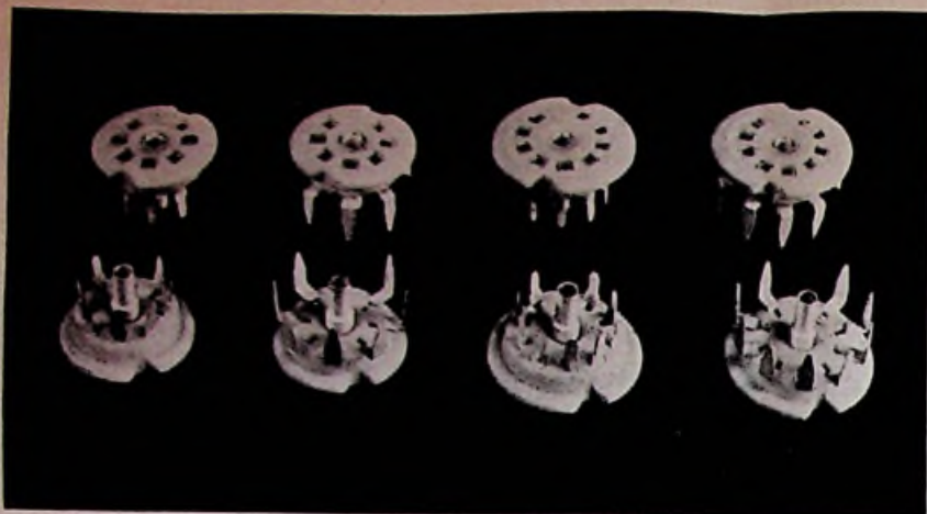
Fig. 4. Keramische buishouders voor gebruik met gedrukte bedrading
