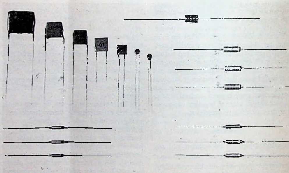
Fig. 1. Miniatuur condensatoren voor transistorschakelingen
